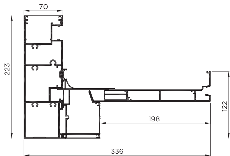
CONJUNTO MONTAJE COMPENSADORES
