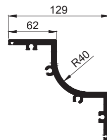
ANGULAR REFUERZO
