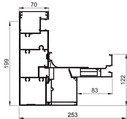
CONJUNTO MONTANTE-COMPENSADORES CON REDUCCIÓN
