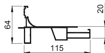
COMPENSADOR 2
