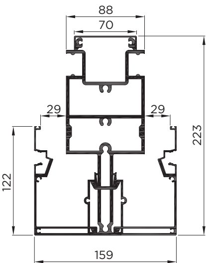
CONJUNTO MONTAJE CENTRAL-CANALES
