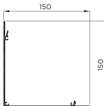
TAPA PILAR
