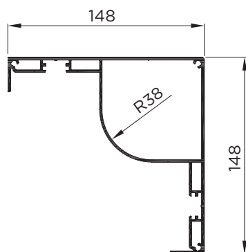
PILAR
