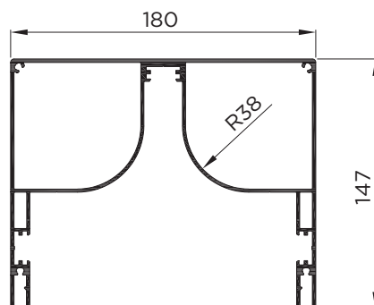
PILAR DOBLE
