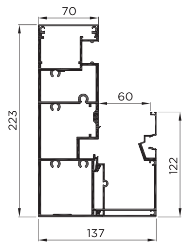
CONJUNTO MONTAJE CANAL
